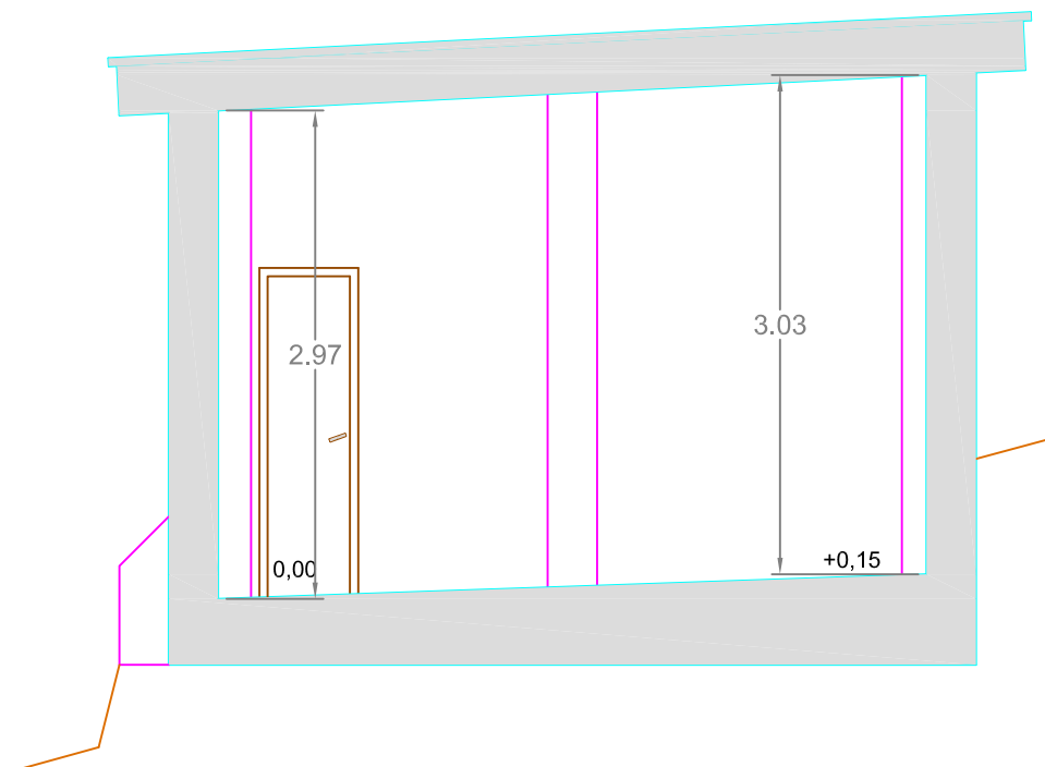
Sección
