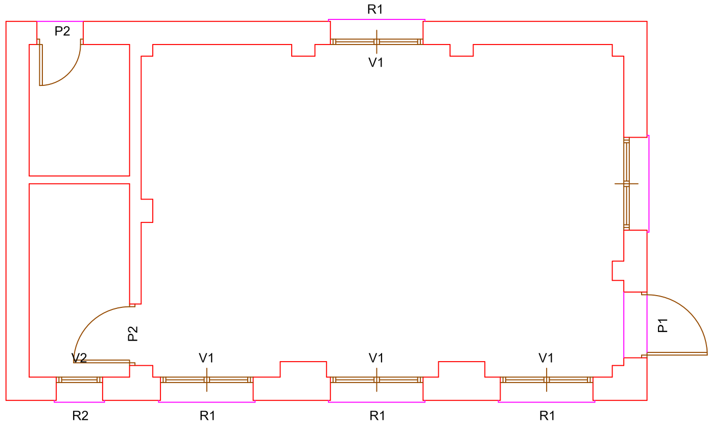
Planta de Instalaciones
