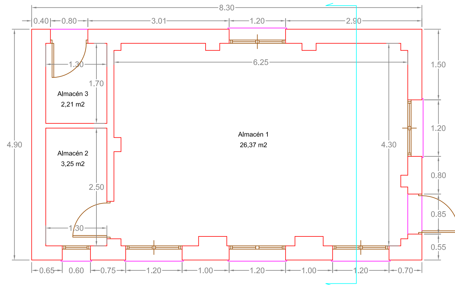
Planta de Cotas y superficies Total superficie construida: 40,67 m2
